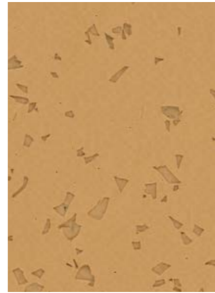
STELLAR - 4039 Pan
