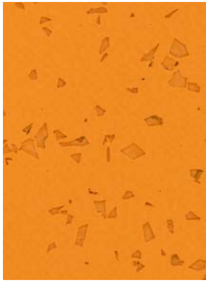
STELLAR - 4163 Flore
