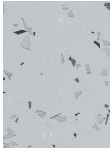
COSMIC - 5721 Fortuna
