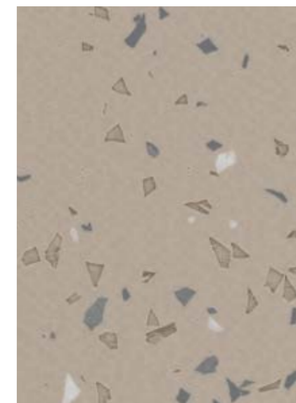
COSMIC - 4369 Egeria
