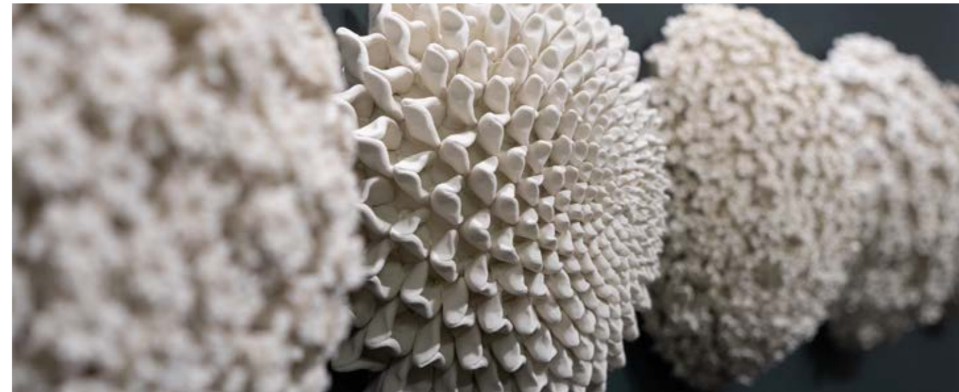
COSMIC - 4036 Vesta
